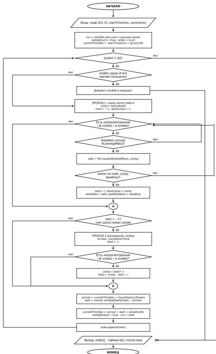
Рисунок 4 – Блок-схема алгоритма ближайшего соседа с временными окнами (NNH-TW)
